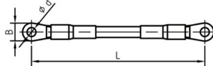
Design B with cable lugs DIN 46234
